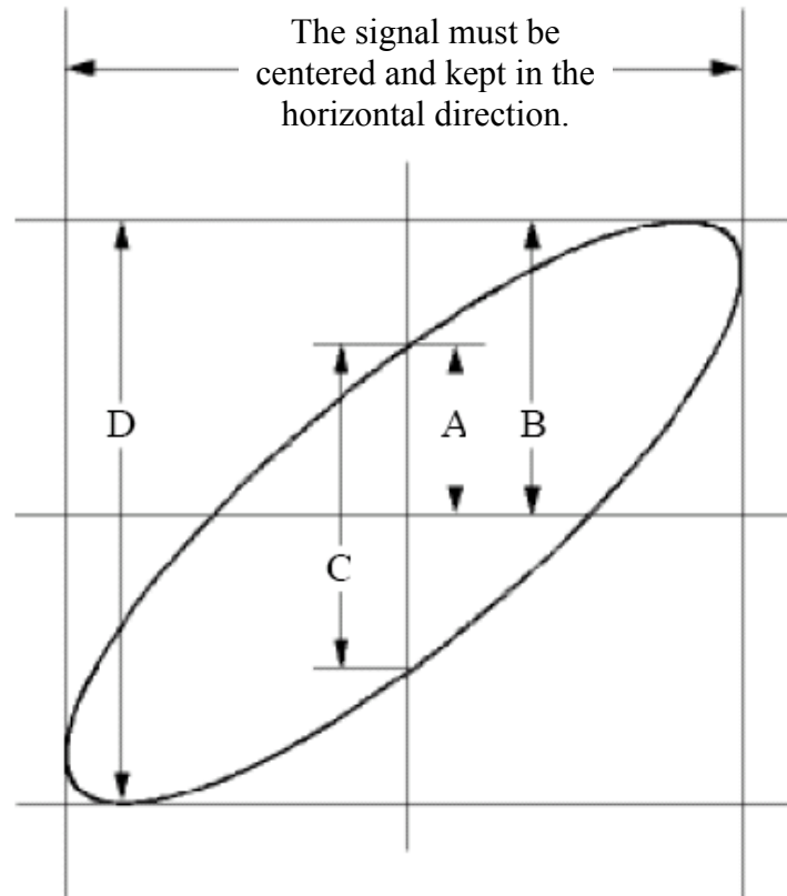
Fig.6-6 Lissajous Graph
