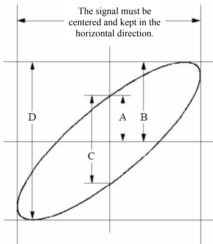
Fig. 95 Lissajous Graph
