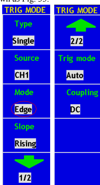
Fig. 33 Edge trigger menu
