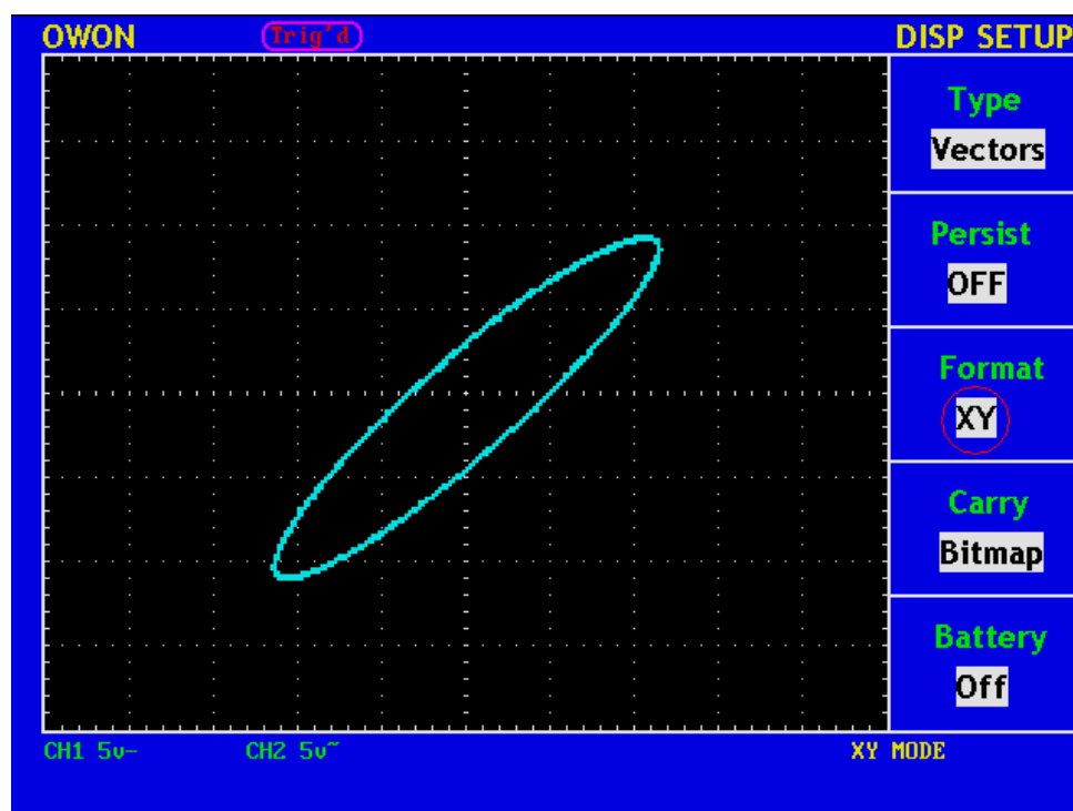
Fig. 49 XY Display Mode
