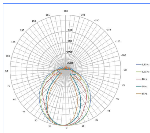
Vertikal Pattern HyperLOG 70 X Serie
