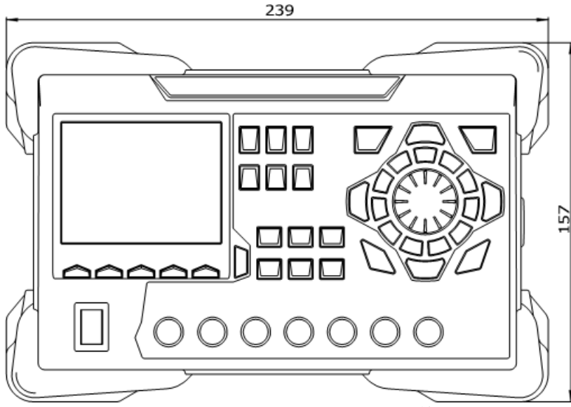
图 1 正视图
