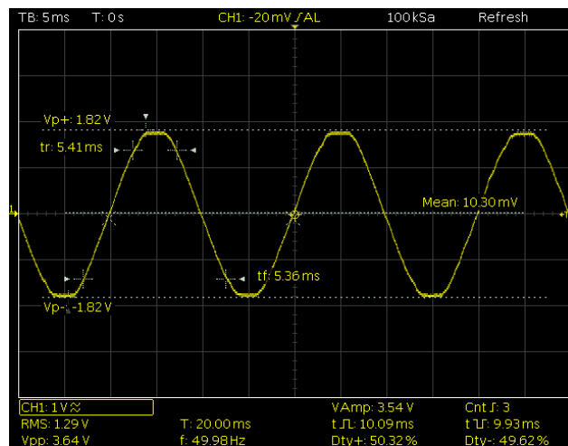
Abb. 6.33: Analog Out Beispiel
