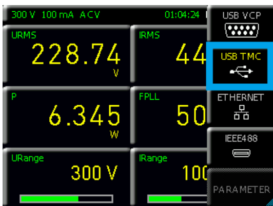
Abb. 10.7: Schnittstellen-Menü
