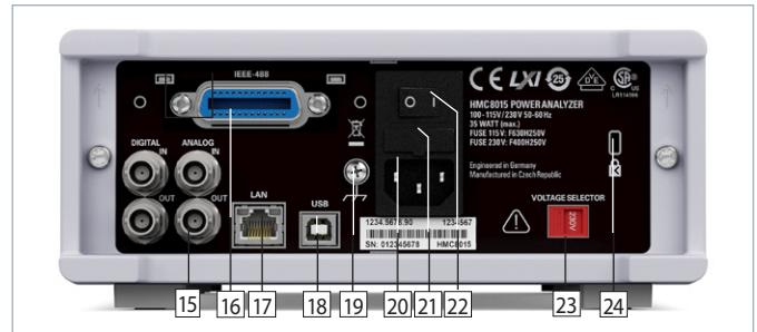
Abb. 2.2: Geräterückseite R&S®HMC8015
