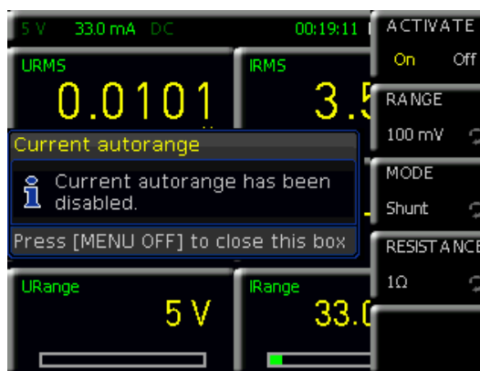
Abb. 4.10: Sensor-Menü
