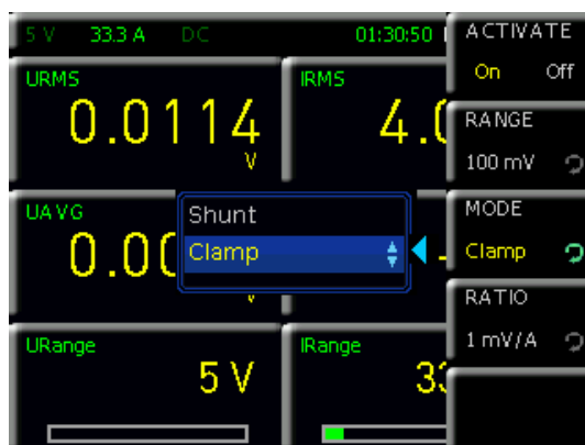
Abb. 4.12: Sensor-Modus
