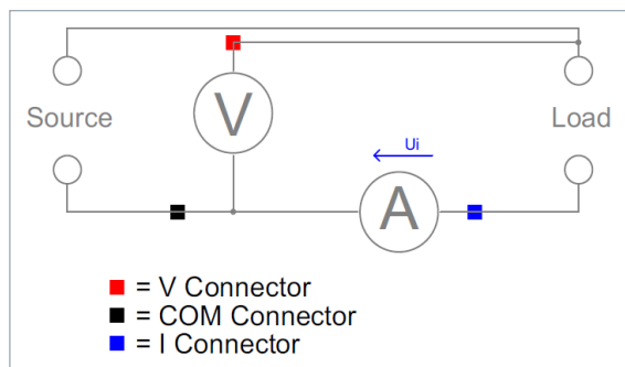
Abb. 4.7: Stromrichtige Messung
