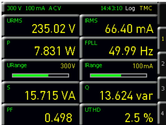
Abb. 6.1: Messwertanzeige R&amp;S®HMC8015
