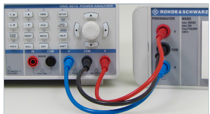
Abb. 4.6: Spannungsrichtige Messung Anschlussbeispiel
