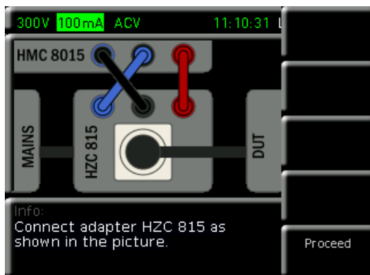
Abb. 6.14: HZC815 Anschlussbeispiel EN 50564
