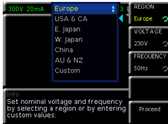
Abb. 6.13: Einstellungsmenü EN 50564
