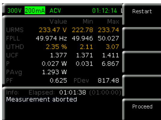
Abb. 6.15: Compliance Test Messbeispiel EN 50564
