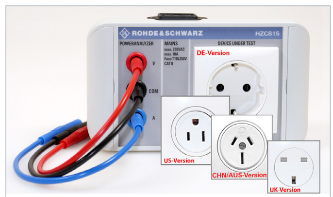
Abb. 4.2: Steckdosenadapter HZC815 DE-, UK-, US- und CHN-Version
