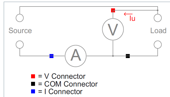
Abb. 4.5: Spannungsrichtige Messung
