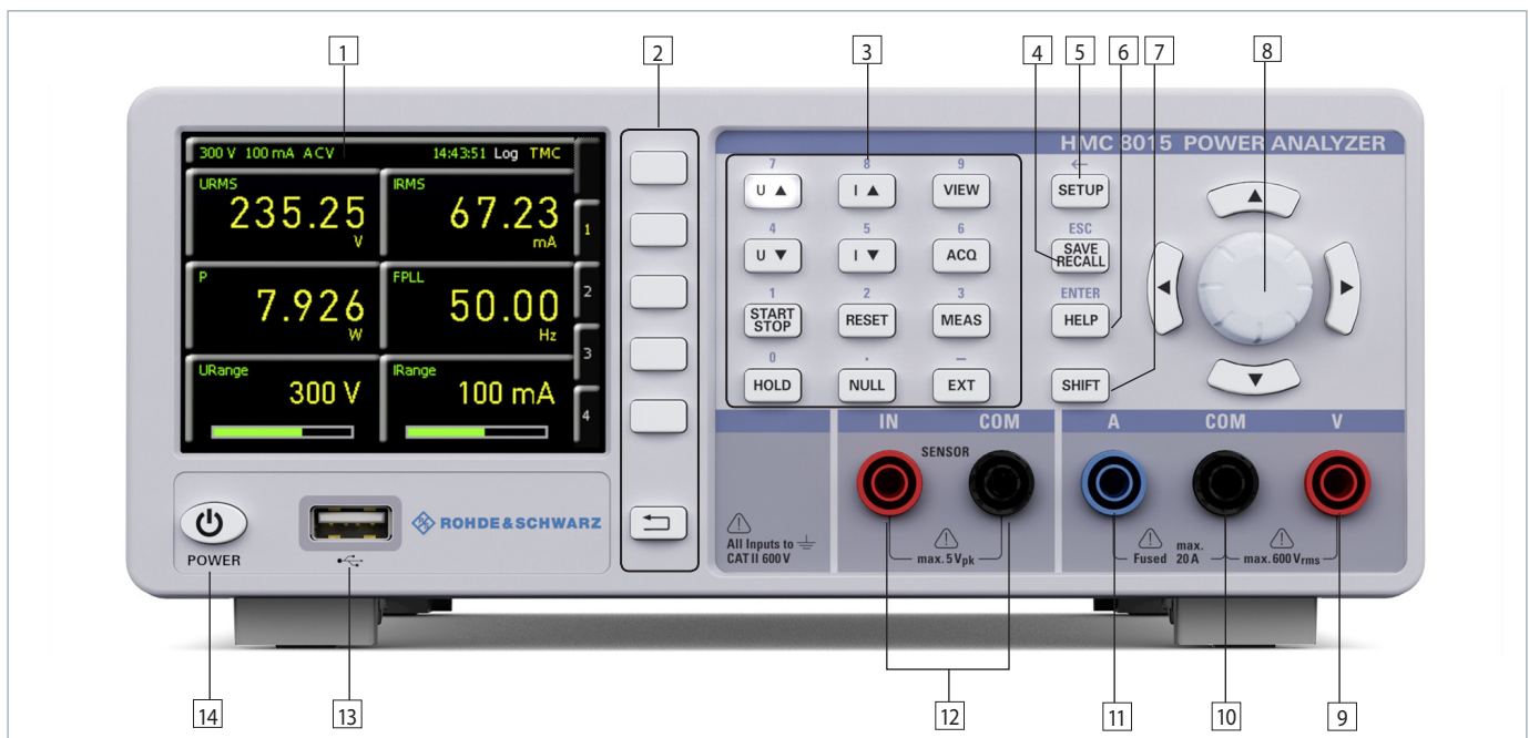
Abb. 2.1: Gerätevorderseite R&S®HMC8015
