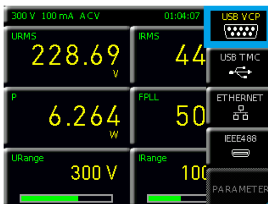
Abb. 10.2: USB-VCP Einstellung
