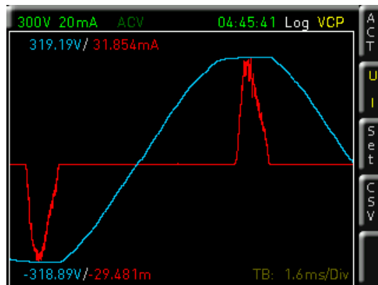
Abb. 6.9: Inrush Modus
