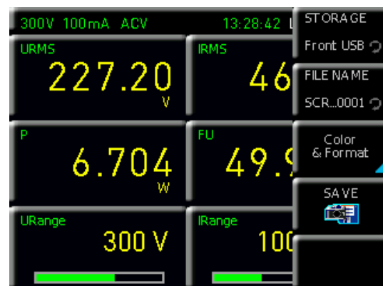
Abb. 8.2: Bildschirmfoto Einstellungsmenü
