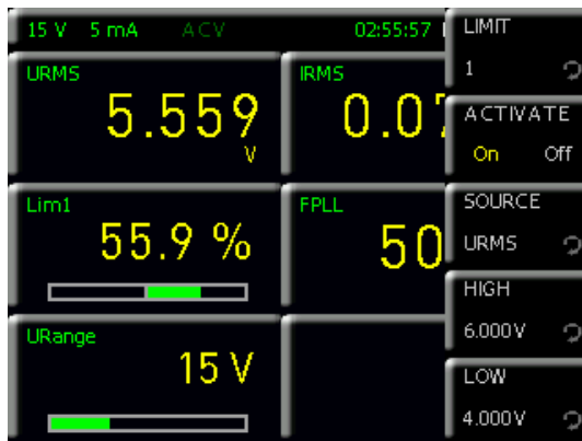
Abb. 6.30: LIMIT-Menü
