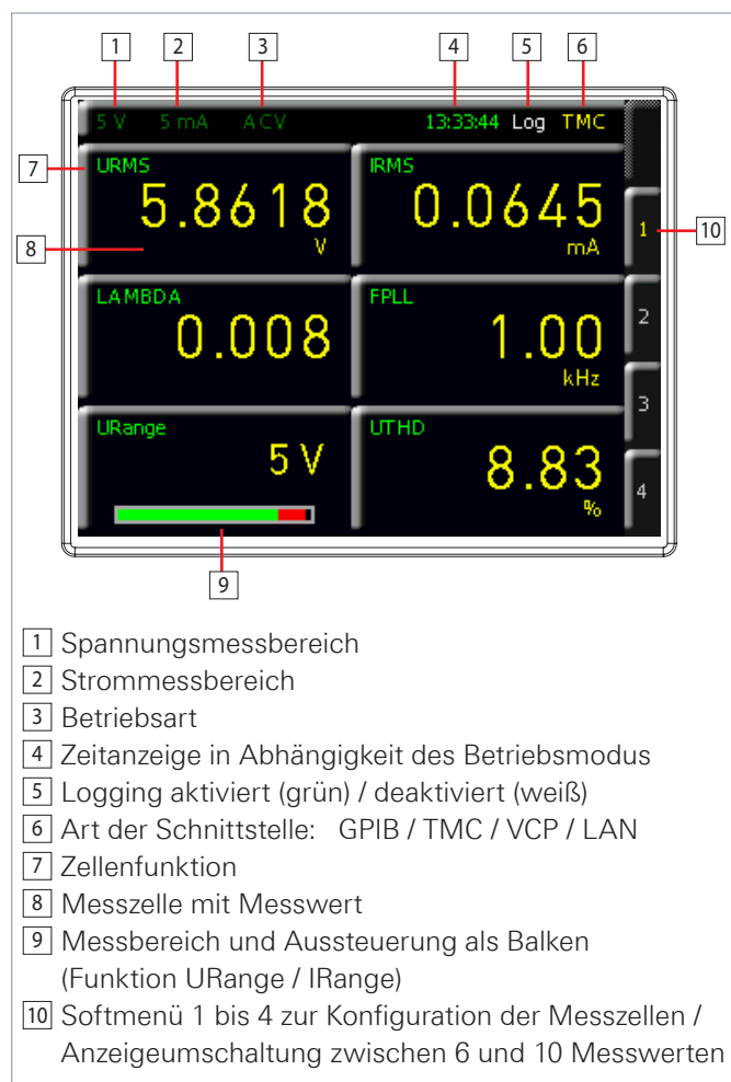
Abb. 5.1: Beschreibung der Bildschirmanzeige
