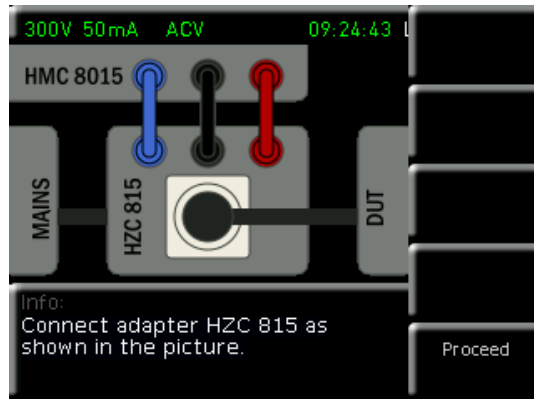
Abb. 6.18: HZC815 Anschluss IEC 61000-3-2
