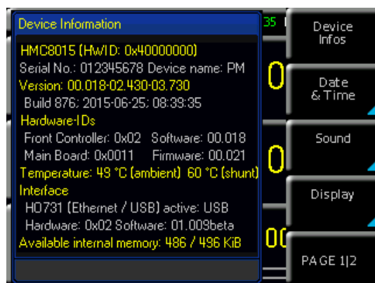
Abb. 9.3: Geräteinformation
