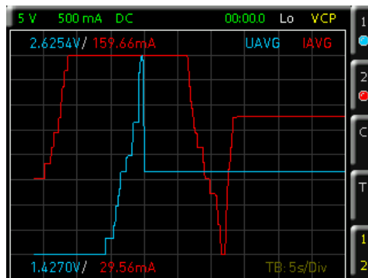
Abb. 6.8: Trendchart Modus
